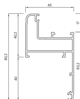
Telaio a "Z" Battuta 40 mm
