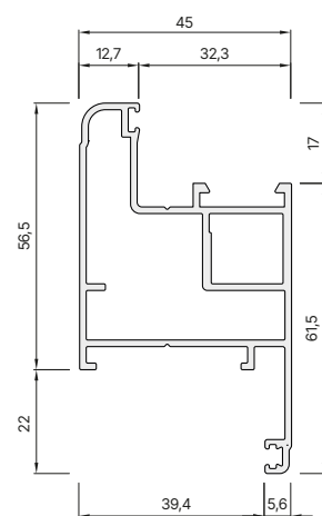
Telaio a "Z" Battuta 22 mm
