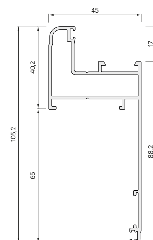
Telaio a "Z" Battuta 65 mm
